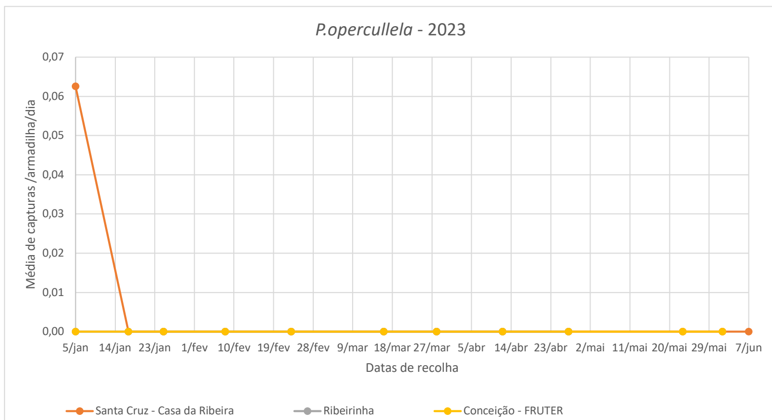
Figura 1- Evolução das capturas médias de adultos por armadilha e por dia de P. operculella , em cada local de monitorização, na Terceira, no ano de 2023.
