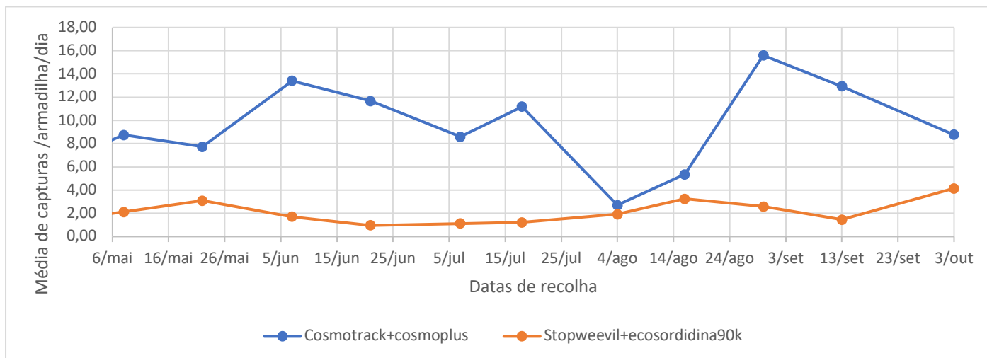
Figura 5 - Evolução das capturas médias /armadilha/dia de adultos de C. sordidus nas 2 armadilhas e 2 atrativos ensaiadas nos pomares de bananeiras na freguesia de São Pedro, no ano 2023.
