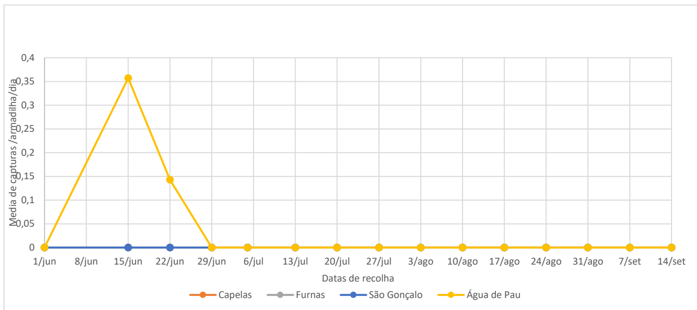
Figura 4 - Capturas de Mythimna unipuncta em Água de Pau, Capelas, Furnas e S.Gonçalo.
