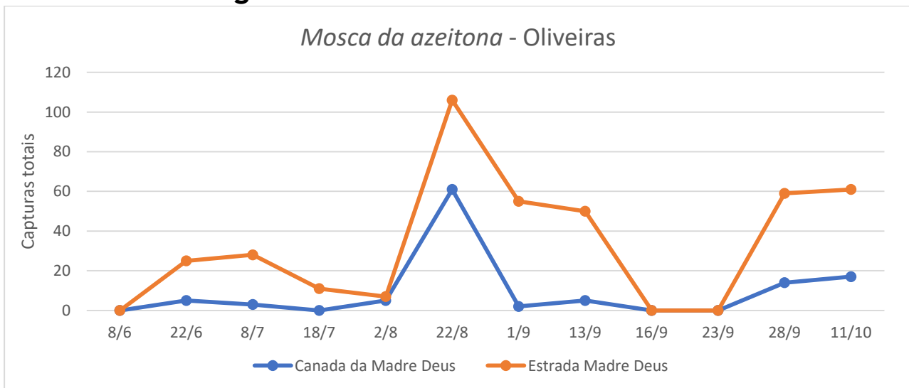
Figura 1- Evolução das capturas de adultos de B. oleae nas 2 parcelas de oliveiras monitorizadas, na freguesia do Porto Martins, no ano 2022.
