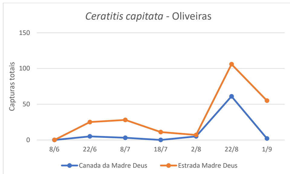
Figura 1- Evolução das capturas de adultos de B. oleae nas 2 parcelas de oliveiras monitorizadas, na freguesia do Porto Martim, no ano 2022.
