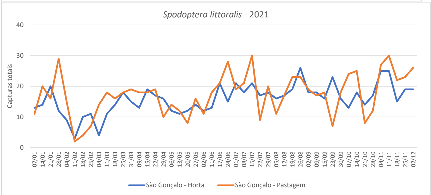
Figura 1 e 1 A- Evolução das capturas de adultos de S. littoralis por armadilha e por dia, nas parcelas monitorizadas nas freguesias de Capelas, Água de Pau e Furnas (acima) e São Gonçalo (abaixo) da ilha de S. Miguel, no ano de 2021.
