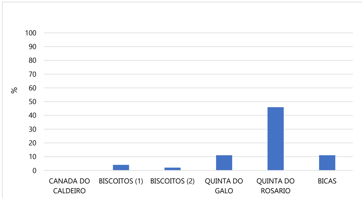
Figura 4 – Distribuição da percentagem de infestação das castanhas por bichado ( Cydia splendana ) nos 6 locais prospeccionados em 2021 (expresso em percentagem com base no número de galerias /fruto).
