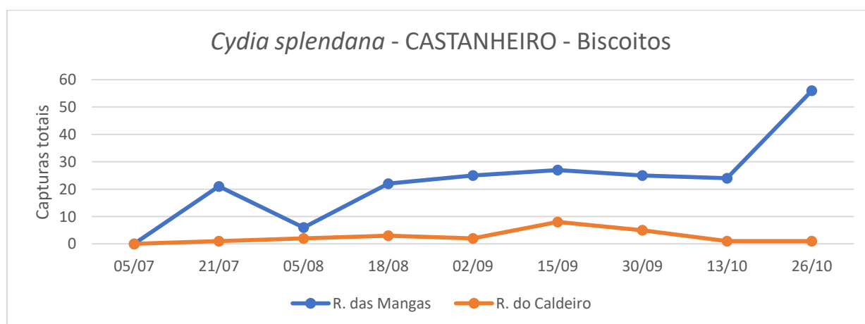
Figura 1- Evolução das capturas de adultos de C.splendana nas parcelas de castanheiro monitorizados, na freguesia de Biscoitos, no ano 2020.
