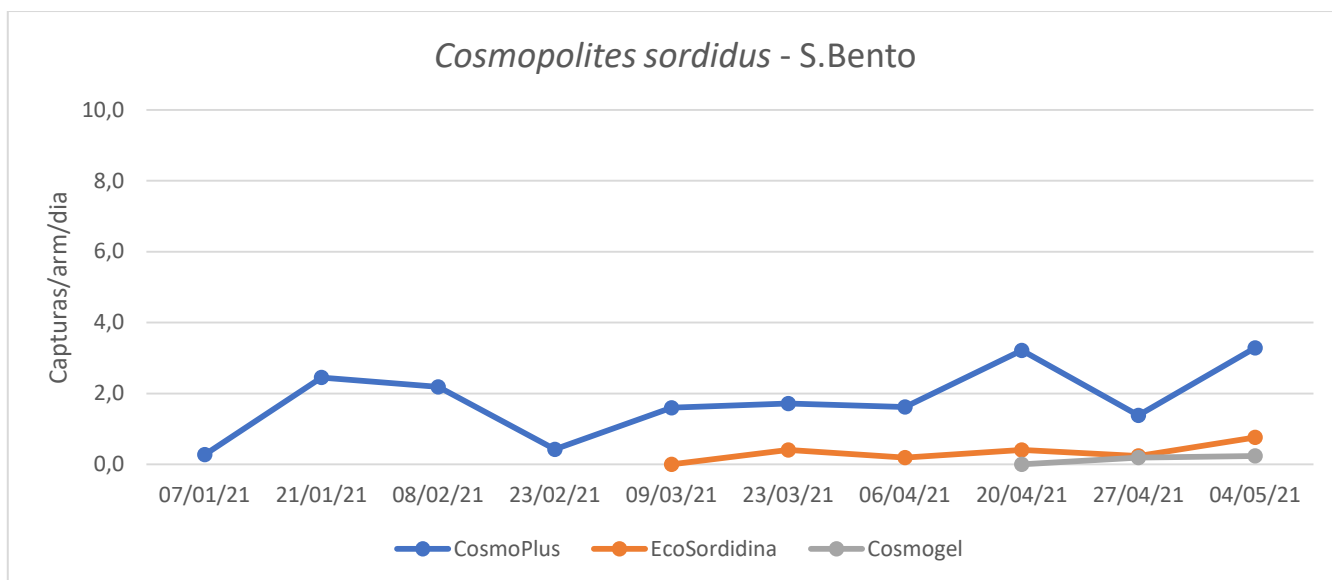
Figura 2 - Evolução das capturas de adultos de C. sordidus nas diferentes armadilhas e atrativos ensaiados nas parcelas de bananeiras na freguesia de S. Pedro e São Bento, no ano 2021.
